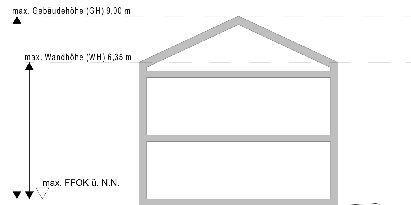
Schemaschnitt 2 - 2 M 1:100
