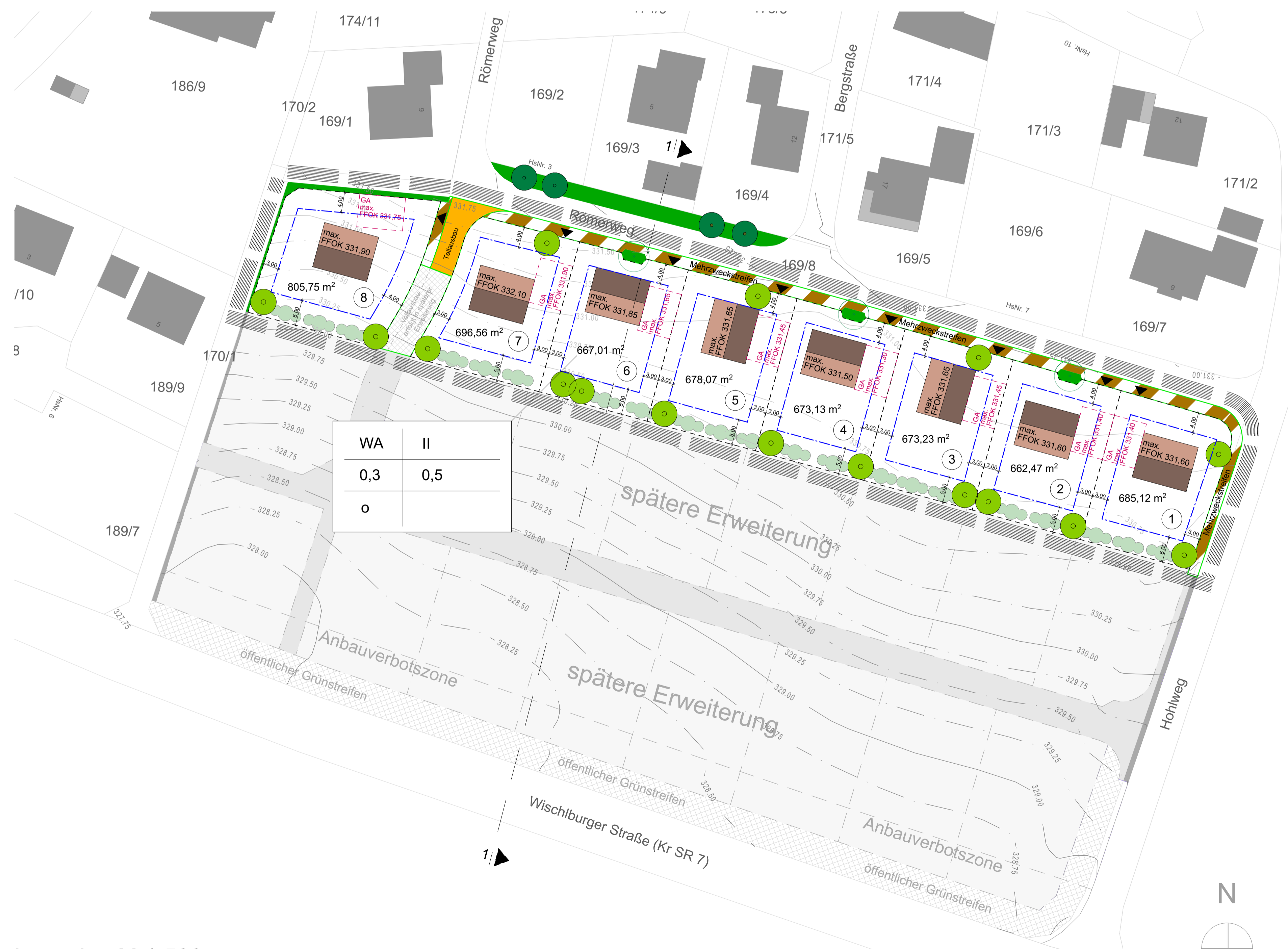
Lageplan M 1:500
